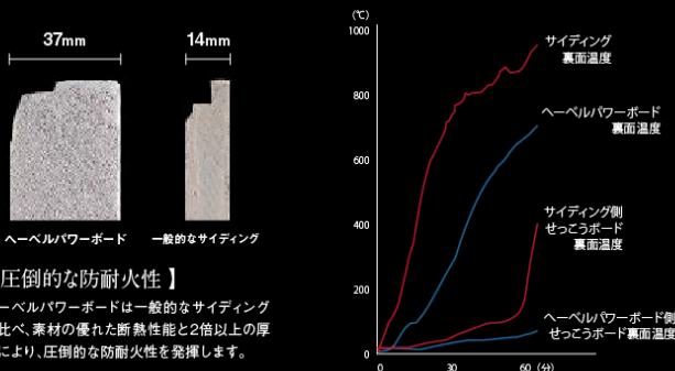
【外壁材裏面と内装せつこうボード裏面の温度変化】
